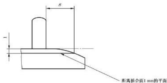
图5 插头边缘示意图
